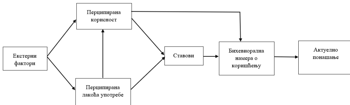
Слика 15: Модел прихватања технологије
