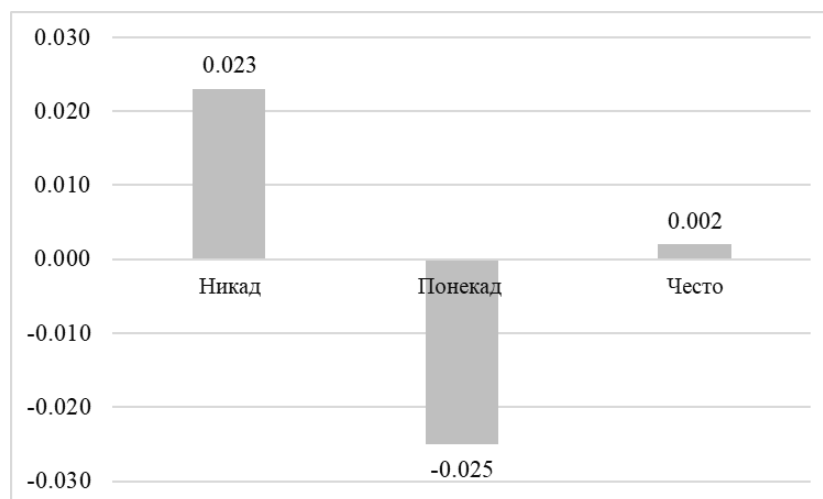
Графикон 2: Парцијалне корисности активности „лајковање”
