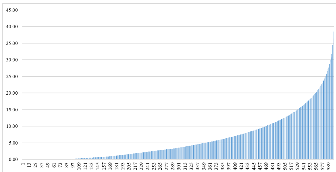
Графикон 6: Коефицијенти дистанци између корака у хијерархијској кластер анализи
