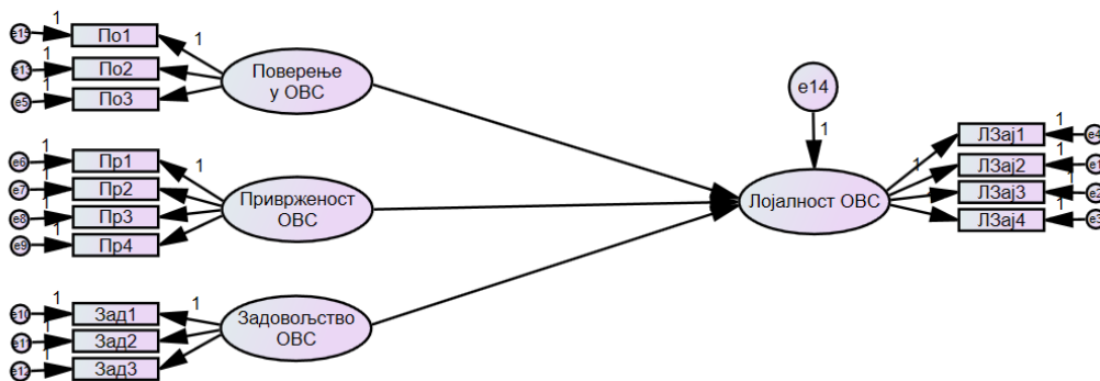
Слика 28: Модел 4 – утицај поверења, привржености и задовољства потрошача ОВС на њихову лојалност ОВС
