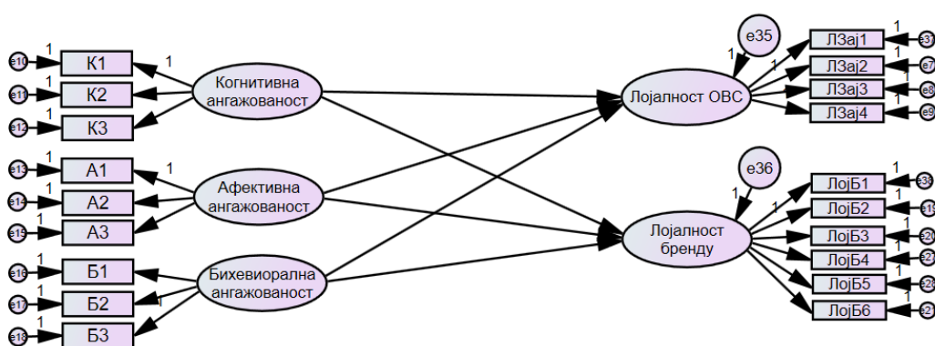
Слика 30: Модел 6 – утицај когнитивне, афективне и бихевиоралне ангажованости на лојалност потрошача заједници и бренду
