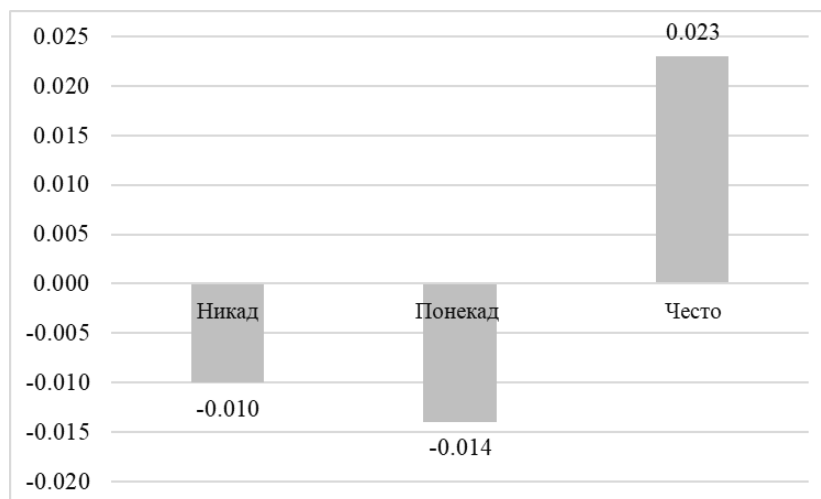
Графикон 1: Парцијалне корисности активности „праћење”
